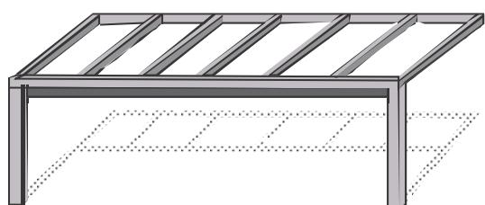
Profil de gouttière Greenline Avec VVK 110/110
